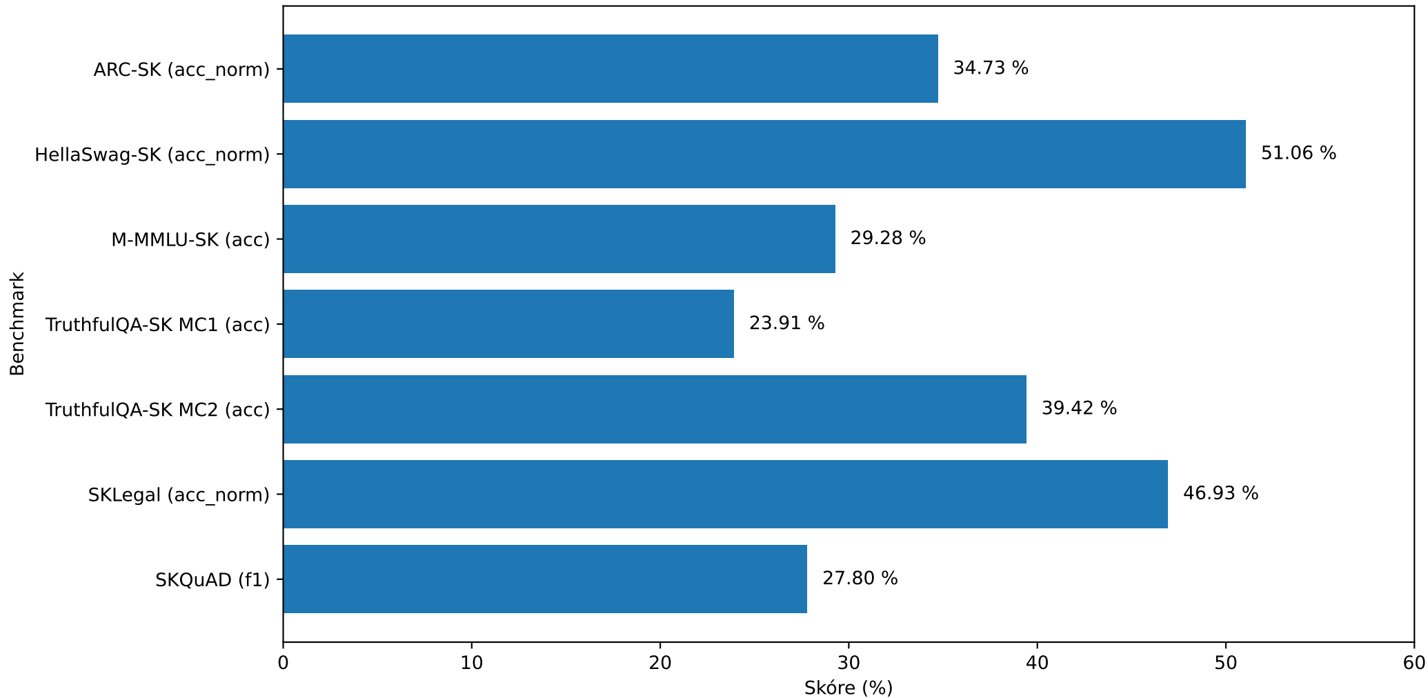
Výsledky lm-evaluation-harness pre PEFT LoRA model
